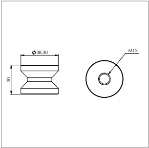
Einschweißgewinde mit M12 Gewinde Für Rundrohre, roh
