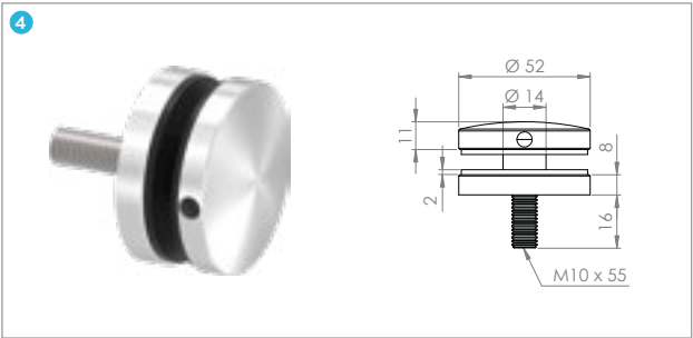
Glaspunkthalter Ø 52 mm
