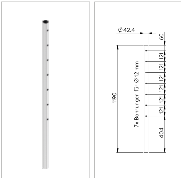
Pfosten, 7x Bohrung einseitig für Ø 12 mm
