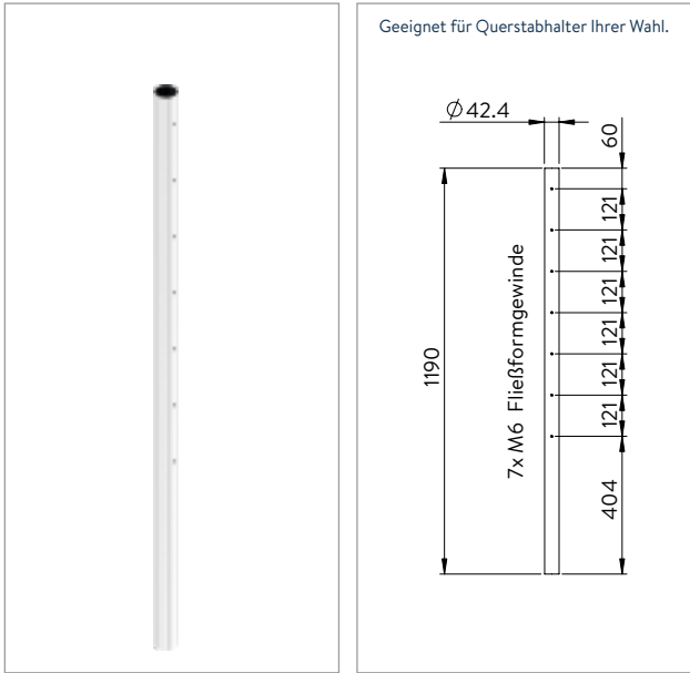
Pfosten, 7x M6 Gewinde einseitig Ohne Befestigung, geschliffen K240
