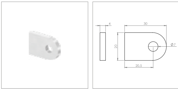
Anschweißlasche 30x20 mm
