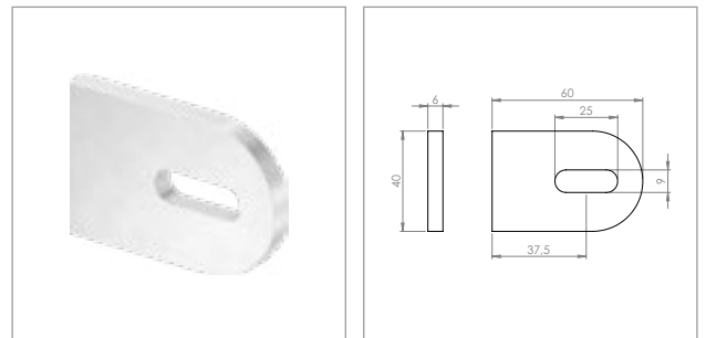
Anschweißlasche 60x40 mm
