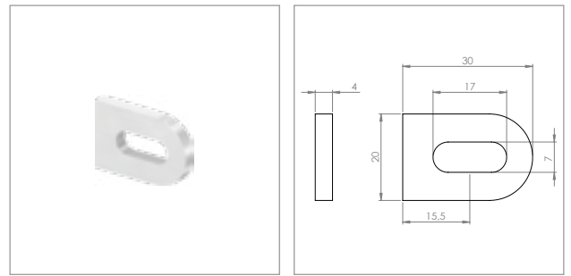
Anschweißlasche 30x20 mm
