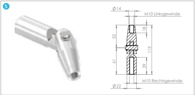
Gelenkverbinder (von Glashalter zu Zugstange)
