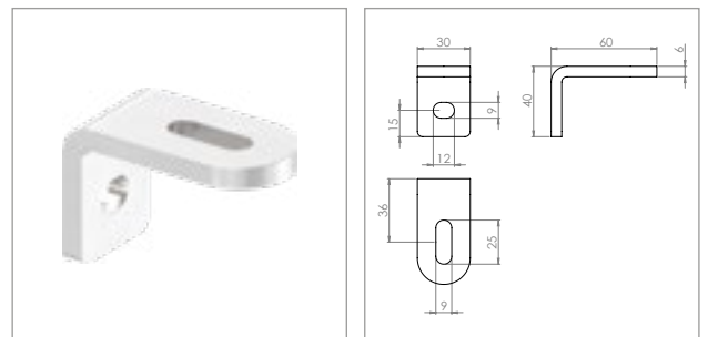
90° Winkellasche 60x40x30 mm
