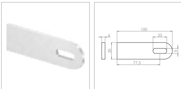
Anschweißlasche 100x30 mm
