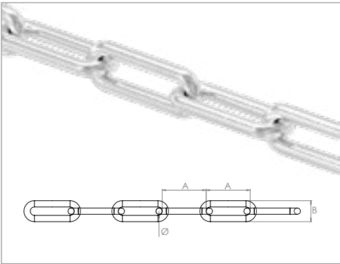
Kette, langgliedrig DIN 763
