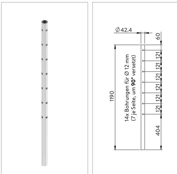
Eckpfosten 90°, 7x Bohrung zweiseitig für Ø 12 mm
