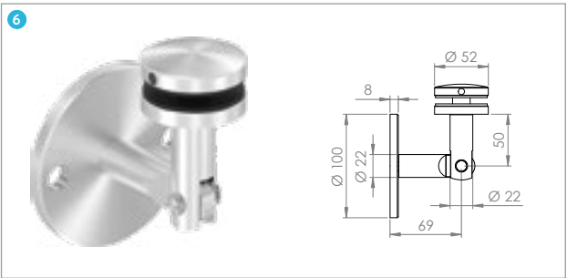
Wandhalter inkl. Glaspunkthalter Ø 52 mm
