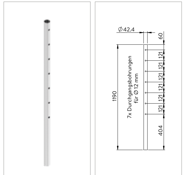
Mittelpfosten 180°, 7x Durchgangsbohrung für Ø 12 mm
