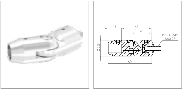
Querstabhalter mit Gelenk (zum Stoßen von vorne)
