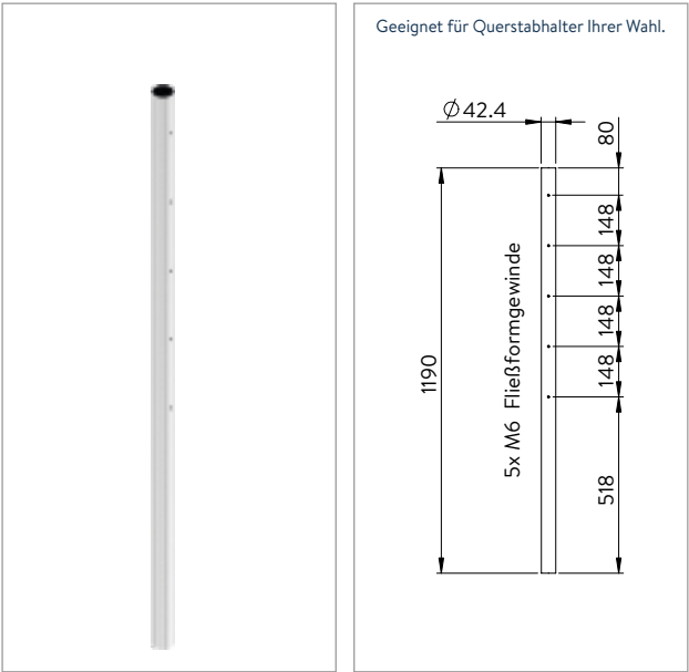
Pfosten, 5x M6 Gewinde einseitig Ohne Befestigung, geschliffen K240
