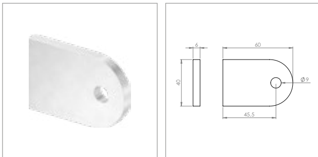
Anschweißlasche 60x40 mm
