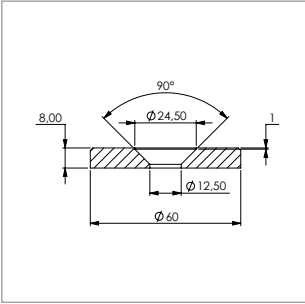
Schraubplatte Ø 60x8mm, mittig gesenkt für M12 Einzel, geschliffen K240
