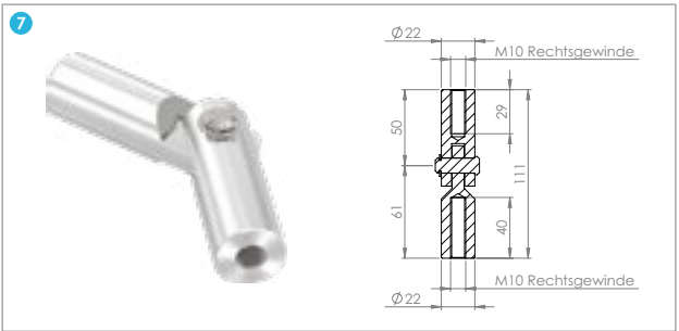
Gelenkverbinder (Ersatzstück für Wandhalter)
