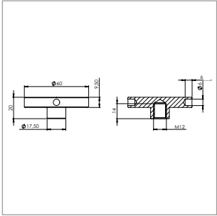
Schraubplatte Ø 60mm mit M12 Gewinde Einzel, geschliffen K240
