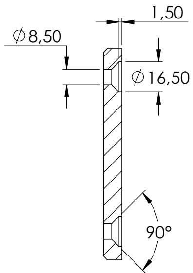
SCHNITT C-C
